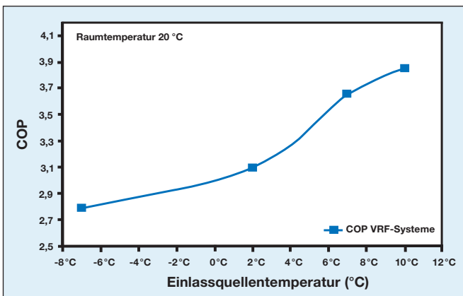
Abb.7 VRF-Systeme: COP Heizen für Auslastung zwischen 10% und 100% nach DIN V 18599 [12] (Bild A.11)
