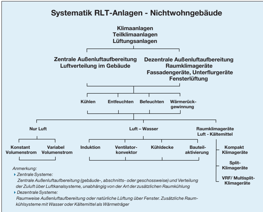
Abb.2 Systematik RLT-Anlagen-Nichtwohngebäude nach [9], Teil 7
