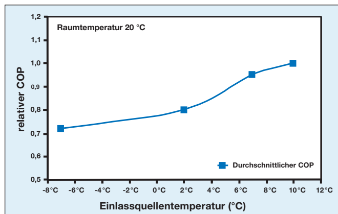
Abb.9 VRF-Systeme: relativer COP Heizen für Auslastung zwischen 10 % und 100 % nach DIN V 18599 [12] (Bild A.11)
