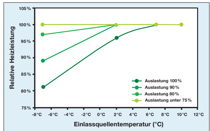
Abb.8 VRF-Systeme: relativer Heizleistungsverlauf nach DIN V 18599 [12] (Bild A.12)
