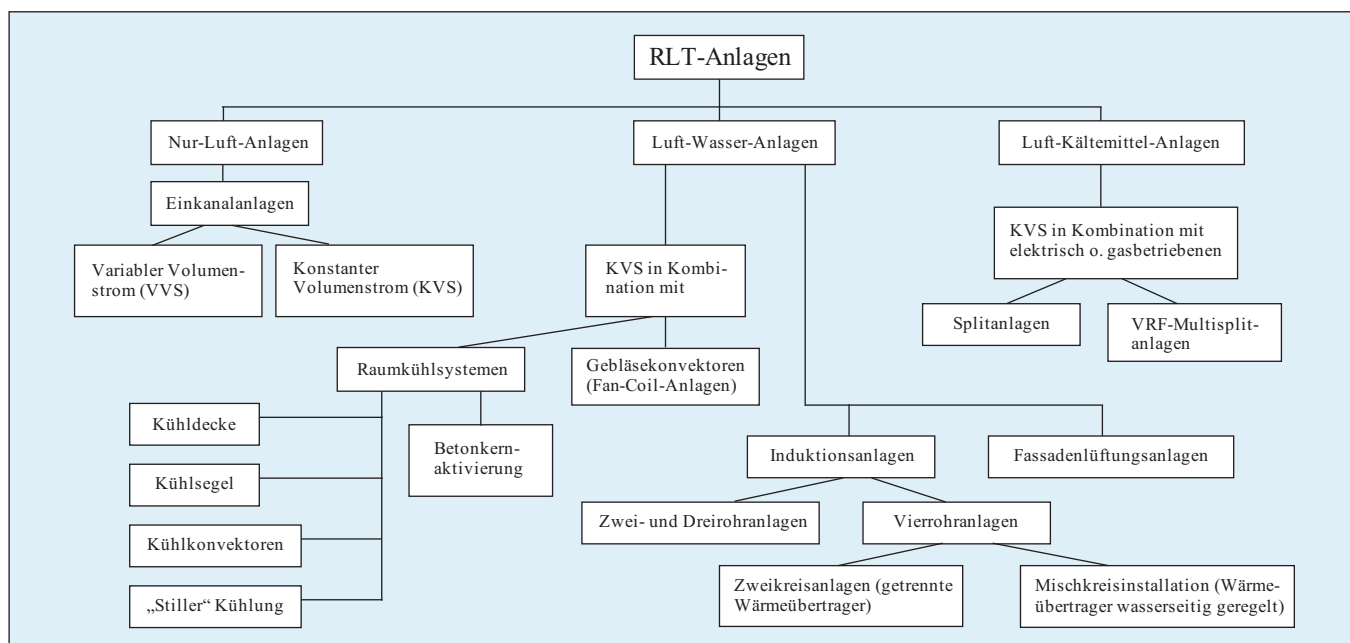
Abb.1 Einteilung der RLТ-Anlagen (erweitert) auf Grundlage von [1]
