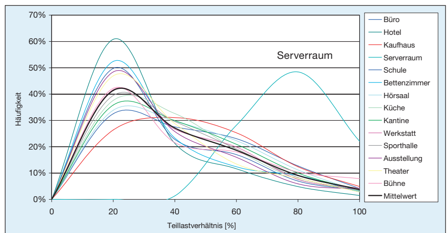
Abb.4 Teillastfaktoren nach DIN V 18599 aus [13]
