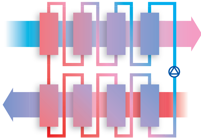
Hochleistungssystem durch Hintereinanderschaltung mehrerer Heiz-/Kühlregister
